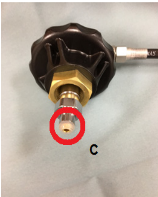
Afbeelding 20: Interface N 2 O-cilinder
