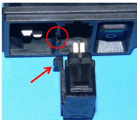
Afbeelding 19: Plaats van geleidingslipje
